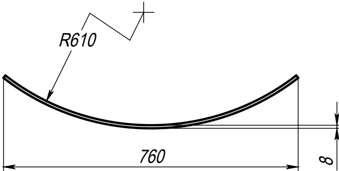
Поз.3 (Хомут)
